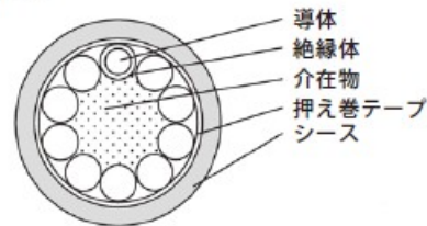
構造図
