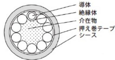
構造図
