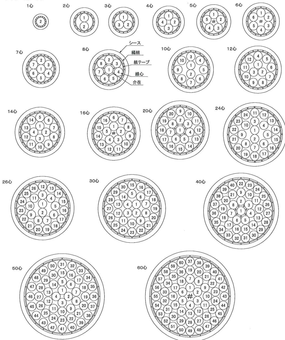
付図：構造図
